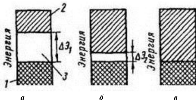
Рисунок 1 - Типовые схемы энергетических уровней электротехнических материалов
